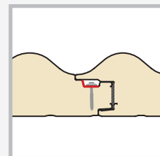
Particolare - Fissaggio nascosto Uni Onda
