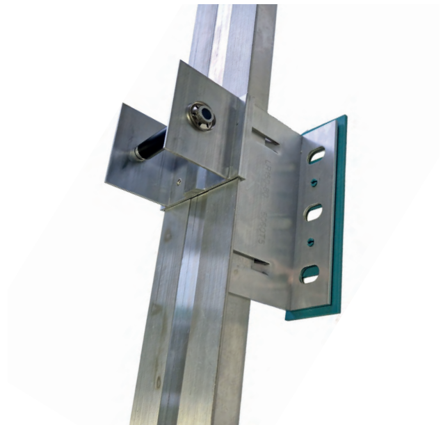
Esempio di installazione profilo Omega.
