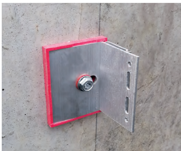
Staffa singola con placca di compensazione in PVC.
